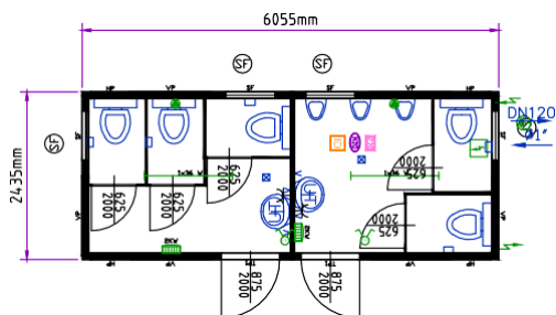
Контейнер-туалет М/Ж 20'
